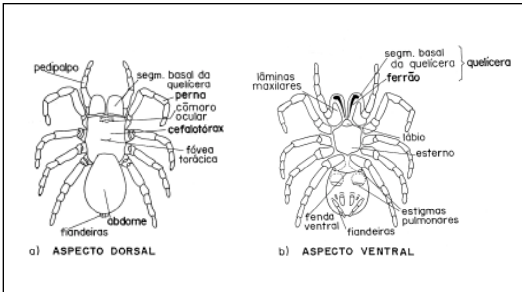
Fig. 37. Morfologia externa das aranhas
